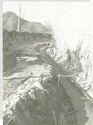
林道改良（新井盗人越線）
