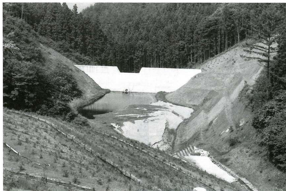
災害防止用の調整池は、過去100年の間に降った最大雨量を想定してつくるため巨大なものに
