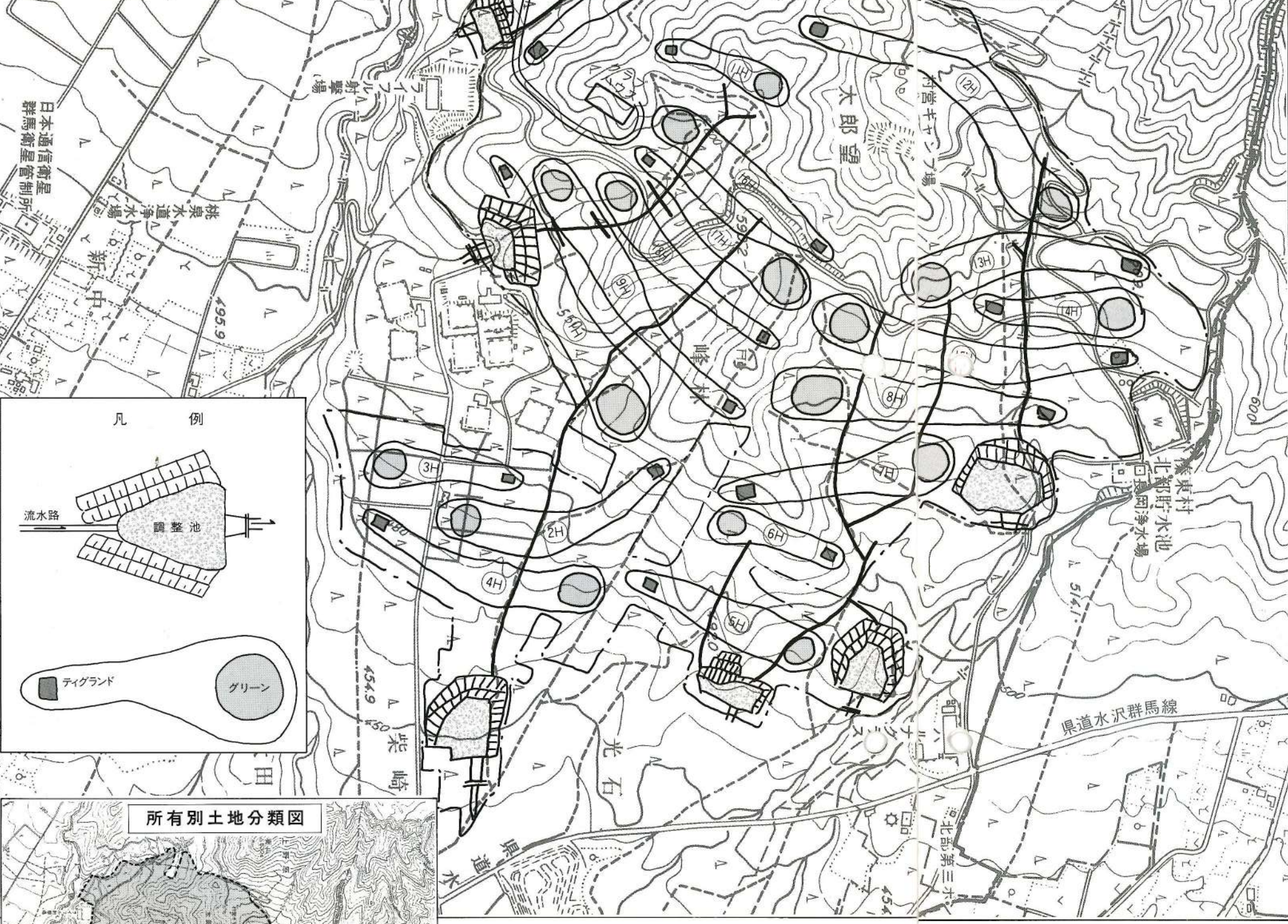
コースおよび調整池配置図
