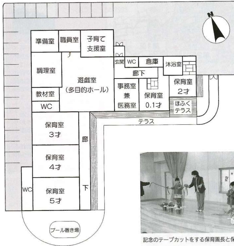
北部保育園平面図
